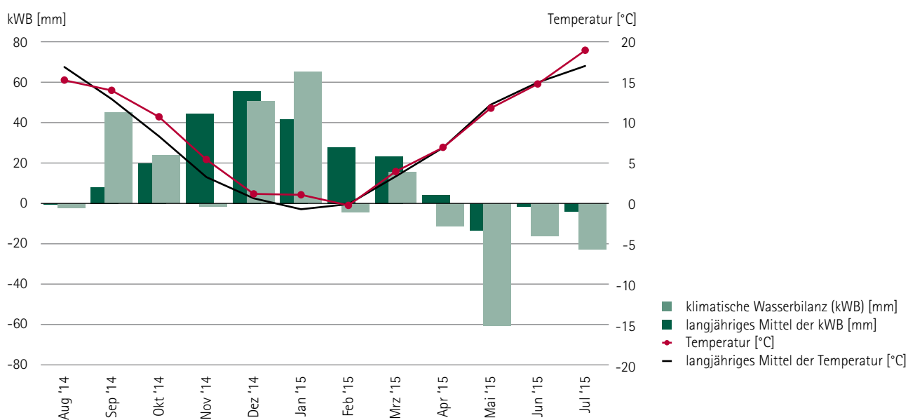
Abb. 6: Witterungsverlauf von August 2014 bis Juli 2015 – Monatsmittel der Lufttemperaturen und die klimatische Wasserbilanz aller Waldklimastationen.
