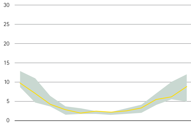
Schwefeldioxid (SO 2 ) – Cunnersdorf [µg/m 3 ]
