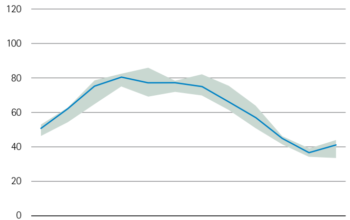
Ozon (O 3 ) – Olbernhau [µg/m 3 ]
