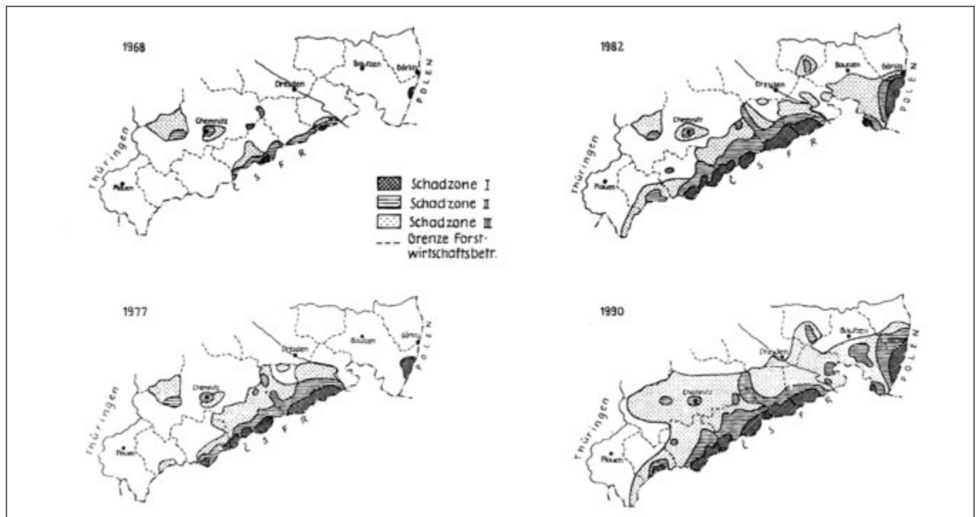
Abb. 21: Schadflächenentwicklung in den sächsischen Fichtenbetrieben. Schadzone I (extreme bis starke Schäden), II (mäßige Schäden), III (leichte Schäden). Aus: Liebold und Drechsler, 1991.
