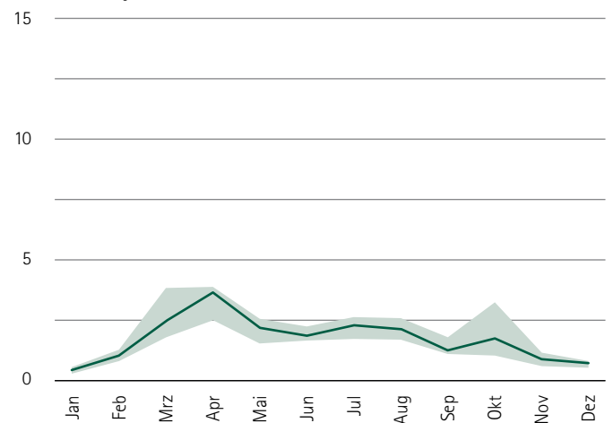
Abb. 20: Mittlerer Jahresverlauf der Schadgase Schwefeldioxid, Ozon, Ammoniak und Stickstoffdioxid für ausgewählte Dauerbeobachtungsflächen (Mediane des Messzeitraumes von 2001 bis 2014 unter Angabe des 25. und 75. Quantils).
