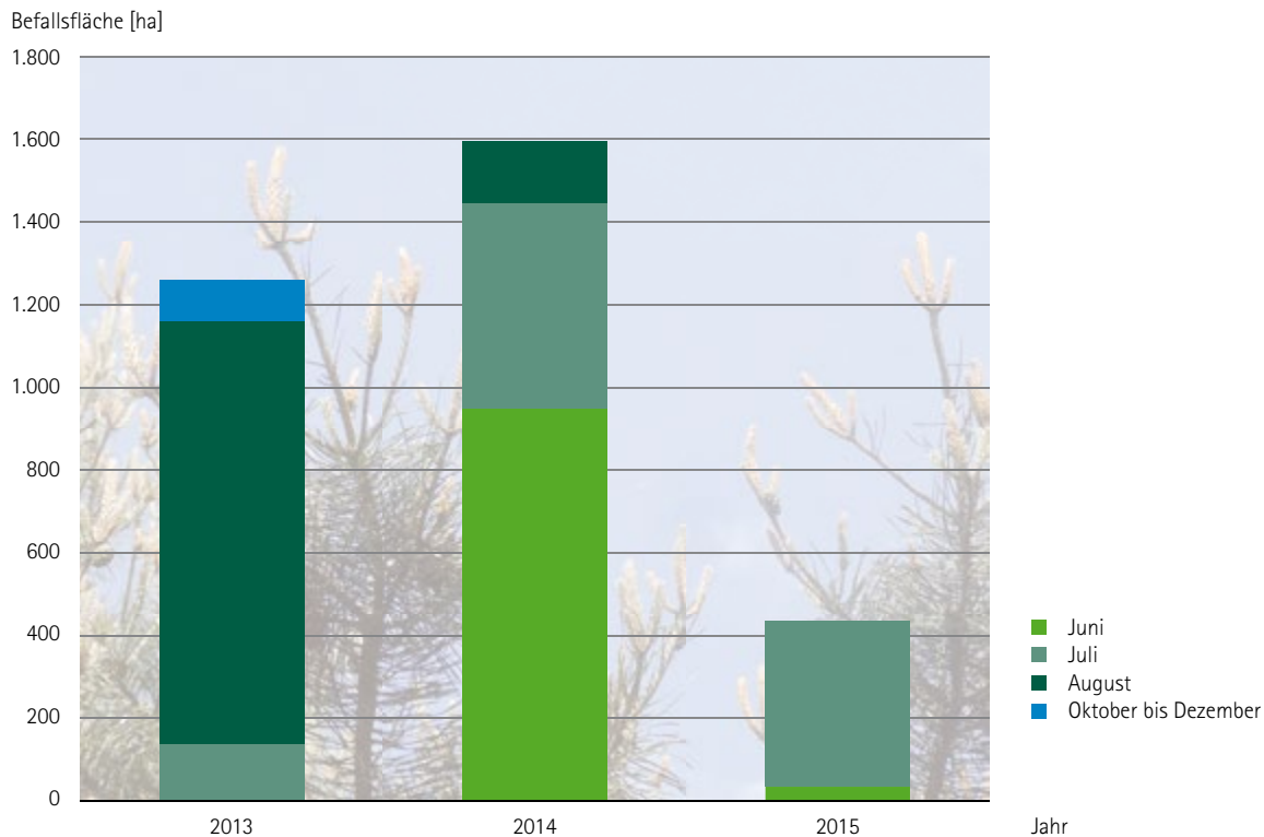
Abb. 39: Von Kiefern Nadelscheidengallmücken befallene Fläche in den Jahren 2013–2015 (nach Meldezeitraum); Hintergrundbild: Vorjahresschadbild im Frühjahr vor dem Maitrieb [Stand: September 2015].
